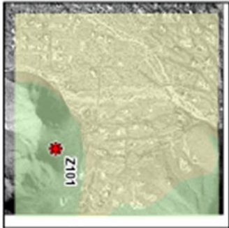
2000 Land Use
